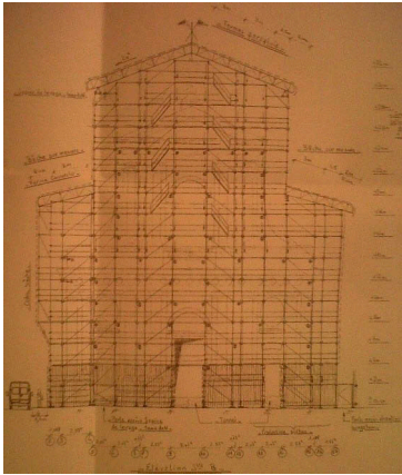
Plan de l'échafaudage
